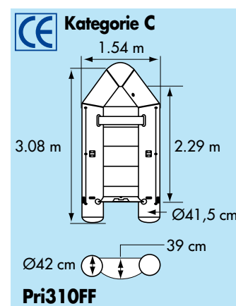
Flacher Boden für Annexe Pri310FF und Pri350FF.
